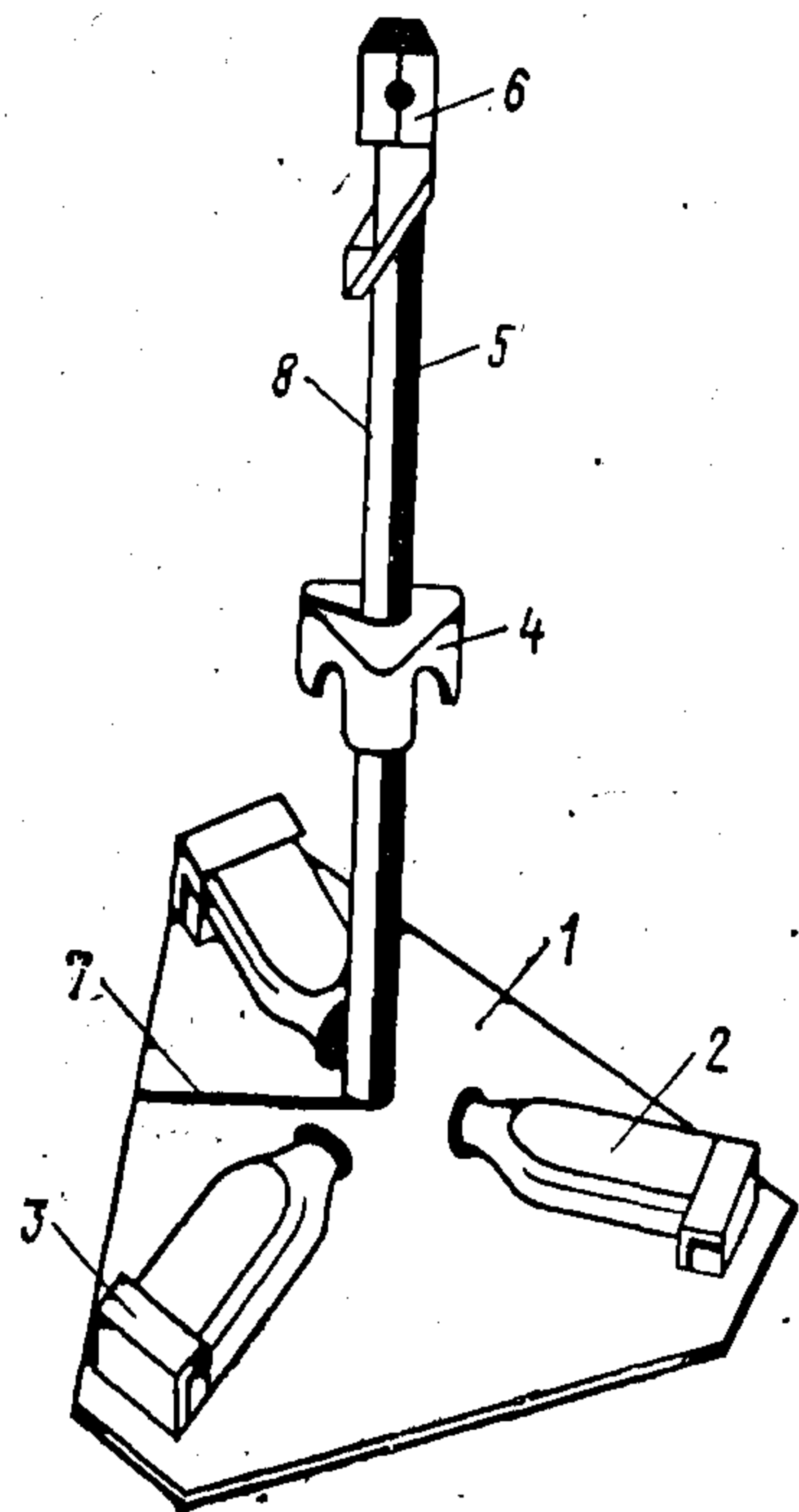
Рис. 34. Продукционный плотик:
