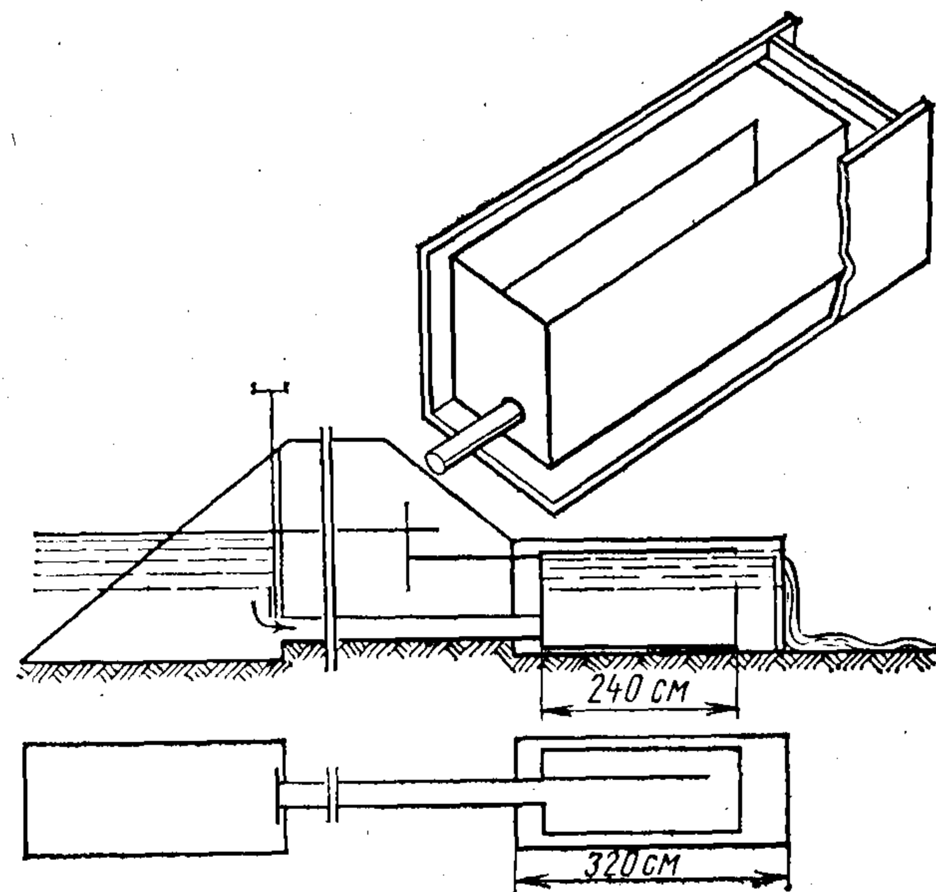
Рис. 48. Мальковый уловитель
