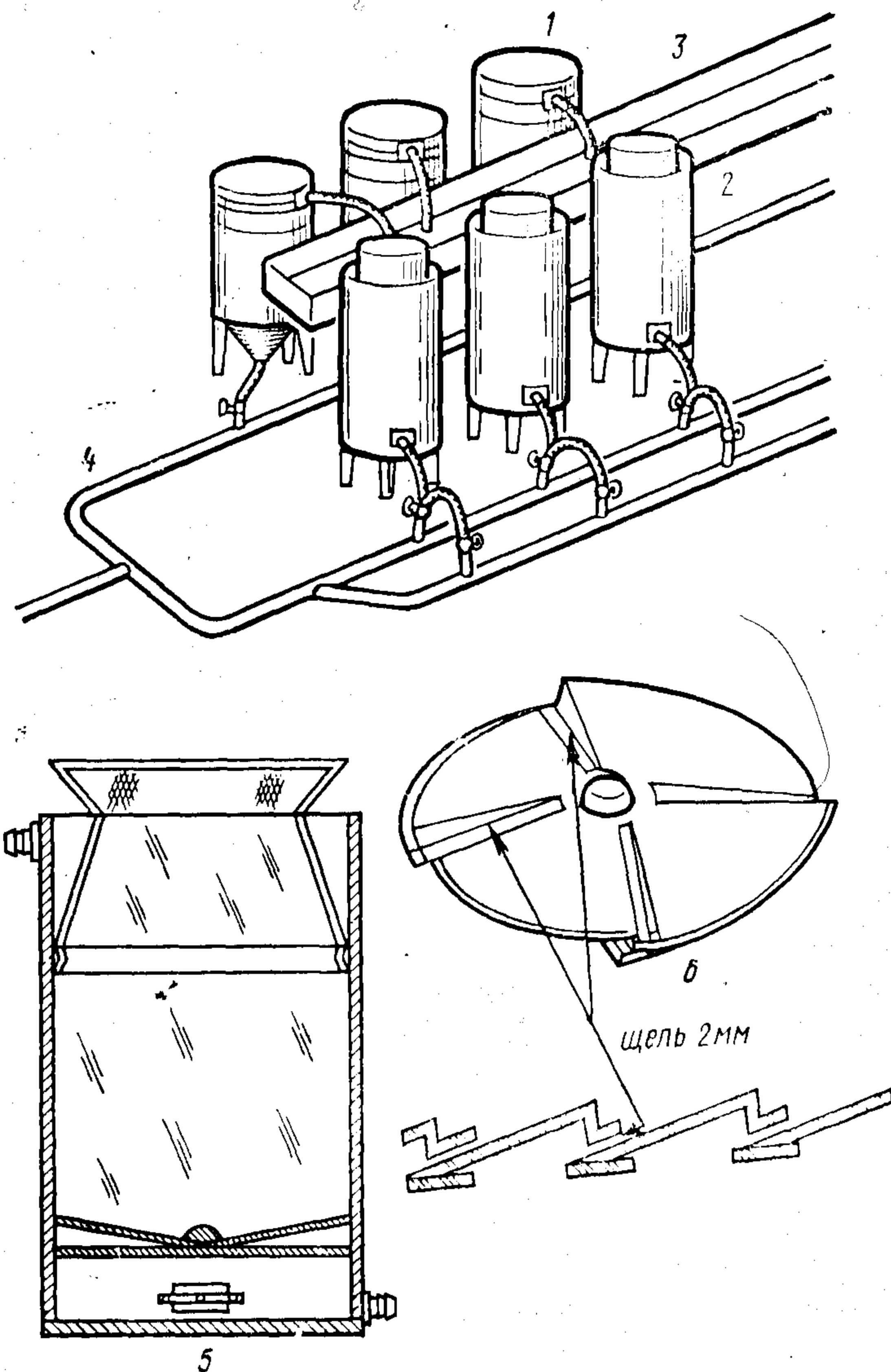
Рис. 52. Аппарат для инкубации икры и содержания личинок рыб:
