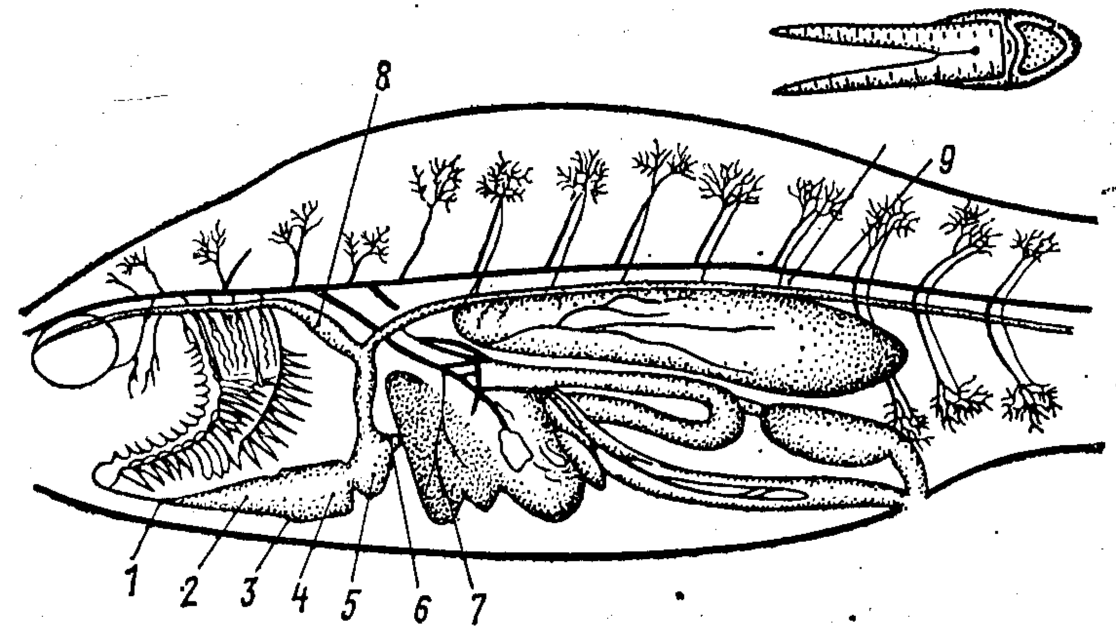
Рис. 3. Схема кровообращения окуня:
