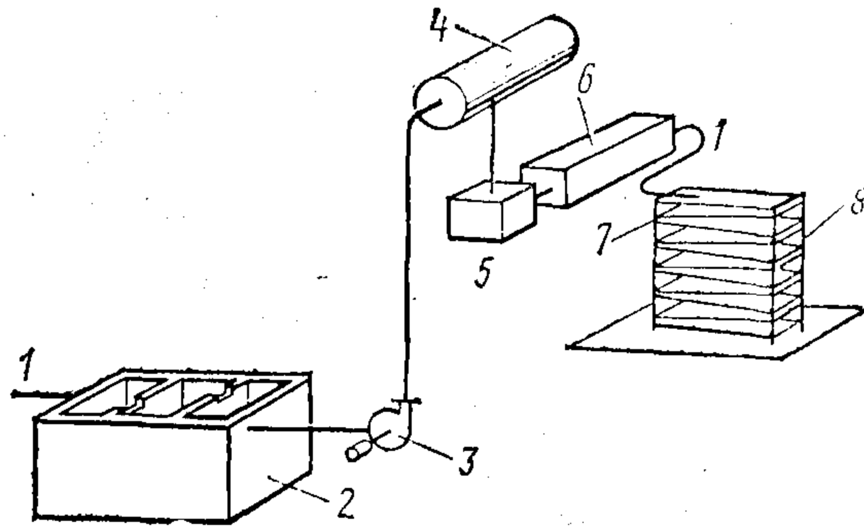
Рис. 54. Лотковый инкубатор:
