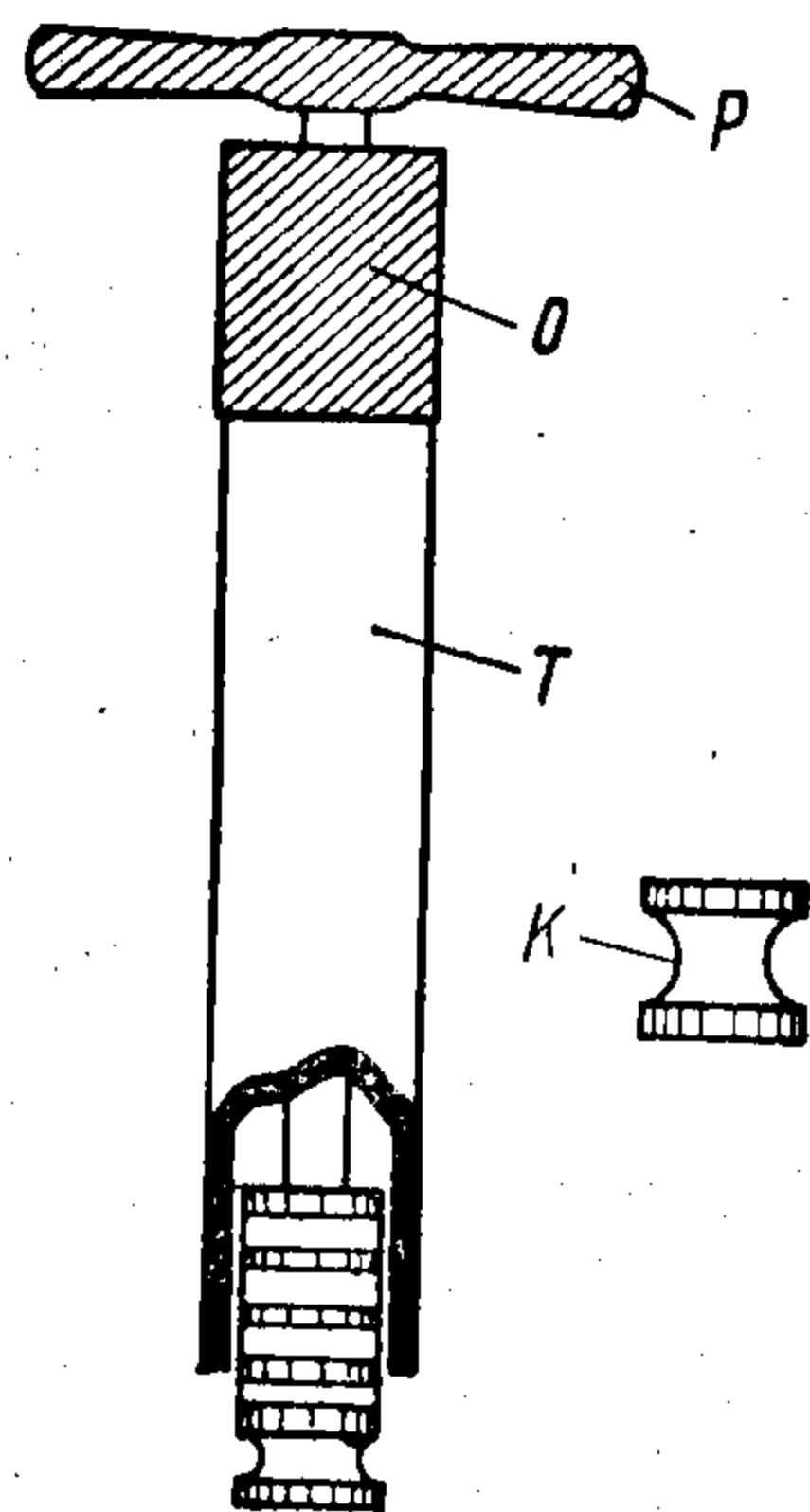
Рис. 36. Штемпель-пипетка
